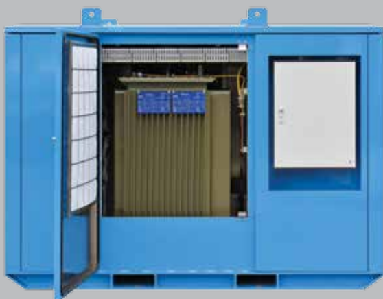
Kompakt transformatorrom med tilgang fra begge sider. Store ventiler i hver dør inn til trafo. Enkelt bytte av ventilasjonsfilter.
