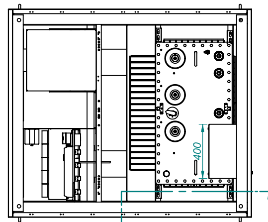
Snitt A-A
